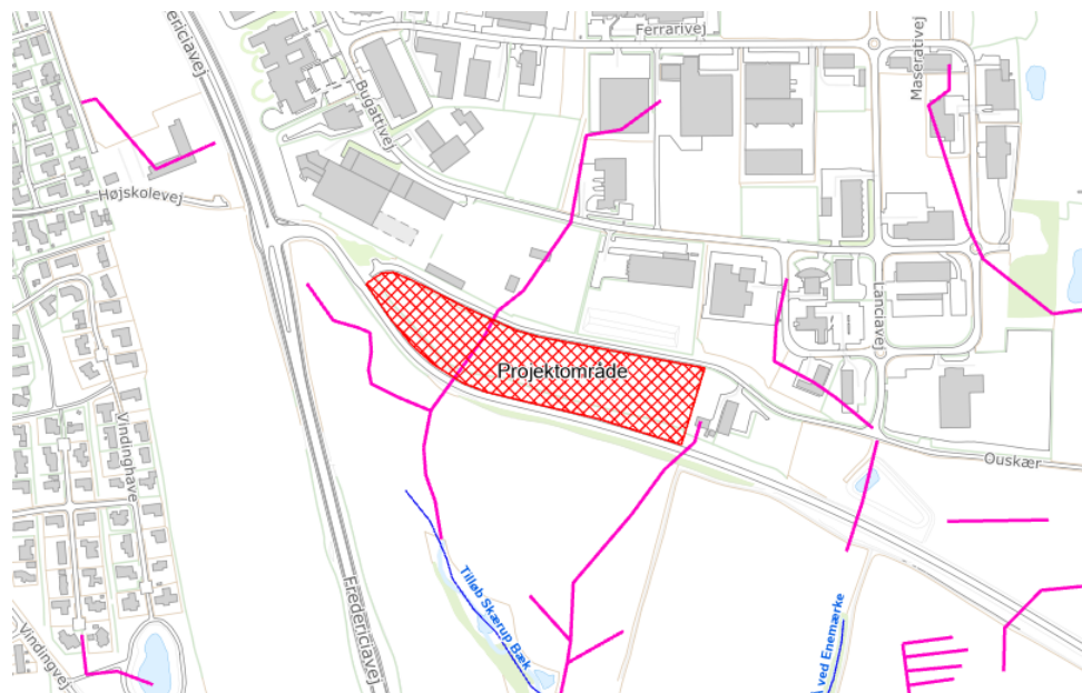
Figur 1 Oversigtskort over projektområde. Lyserøde linjer viser hoveddrænet. Blå linjer er offentlige vandløb.
