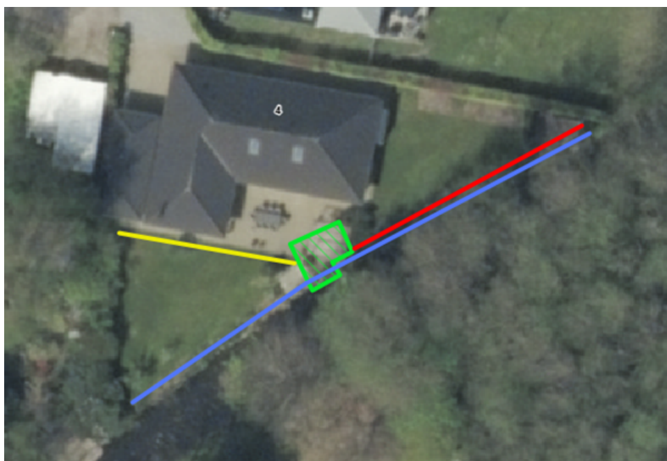
Figur 1: Luftfoto med indtegnert placering af brinksikring (blå), dige (rød), terrasse (grøn) og mur (gul).
