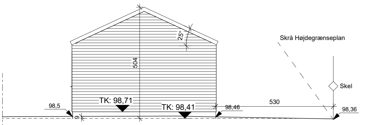
Myn Facade mod øst - vognly
