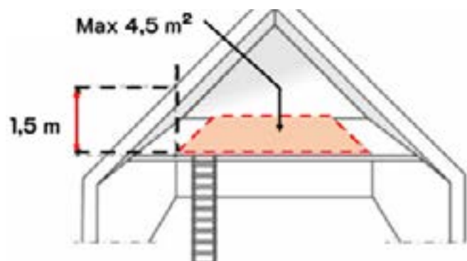
Figur 14. Hems. Her vist hvor den står i åben forbindelse med det rum den er indbygget i.
