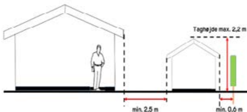
Figur 17. I lodzonen er småbygninger tilladt en maksimal højde på 2,2 meter. Afstand mellem bygninger skal være 2,5 meter. På illustrationen er tagudhæng på begge bygninger mere end 0,5 meter og derfor måles afstanden fra tagudhængets yderste afgrænsning.
