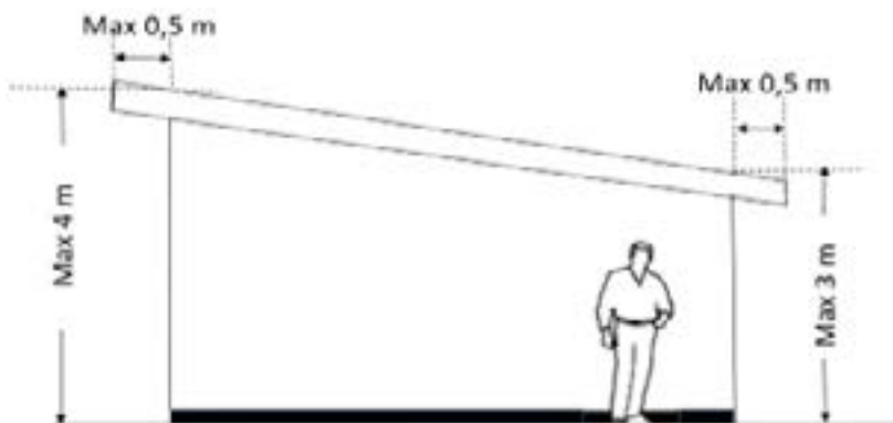
Figur 16. De maksimale facadehøjder på et hus med ensidig taghældning.
