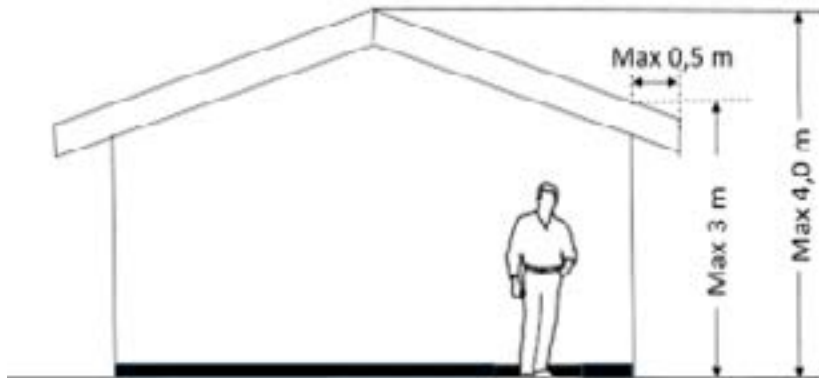
Figur 15. Hus med saddeltag. Den maksimale højde er 4,0 meter og den maksimale facadehøjde 3,0 meter.
