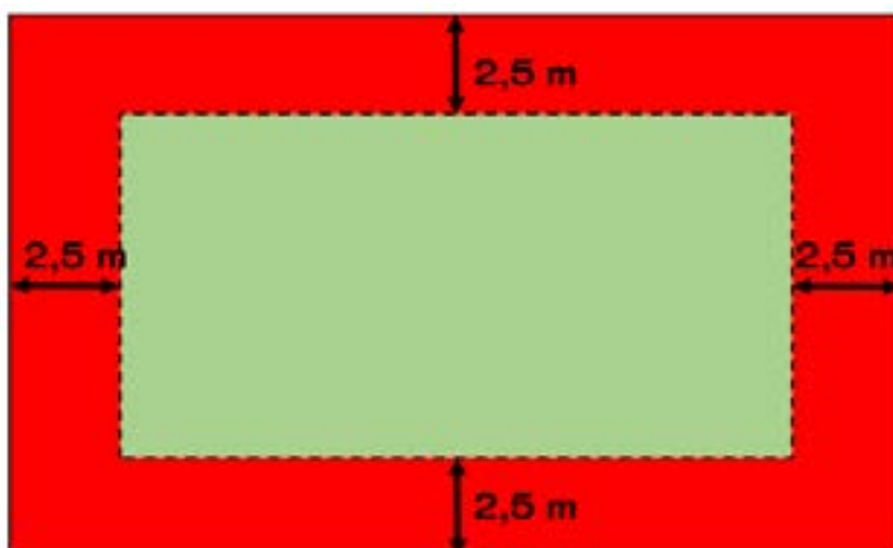
Figur 10. Lodzonen er vist med rødt. Lodzonen måles fra havelodsskel (fastsat ved hækstammen) og 2,5 meter ind på havelodden.
