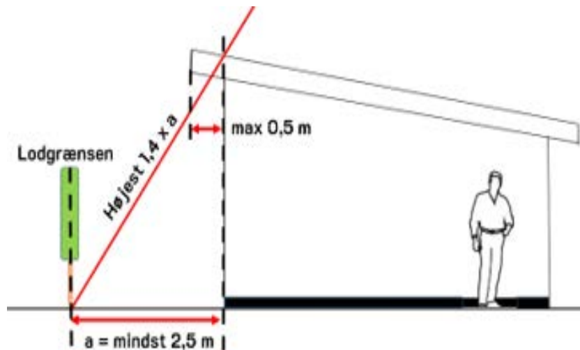
Figur 13. Den maksimale højde på kolonihavehuset beliggende 2,5 meter fra havelodsskel, er 3,5 meter. Tagudhæng op til 0,50 meter kan være i lodzonen.
