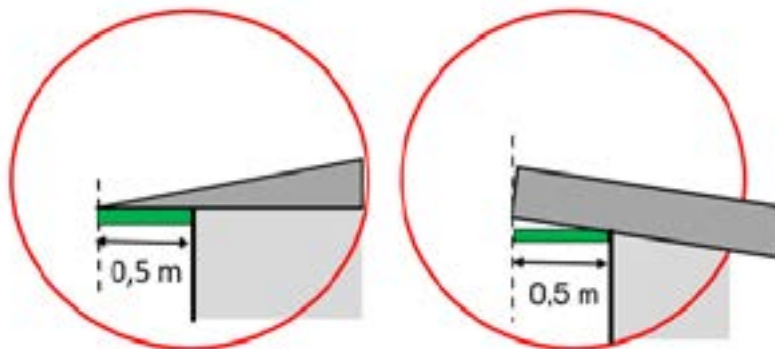
Figur 12. Tagudhæng målt fra henholdsvis bygning med saddeltage og bygning med ensidig taghældning.
